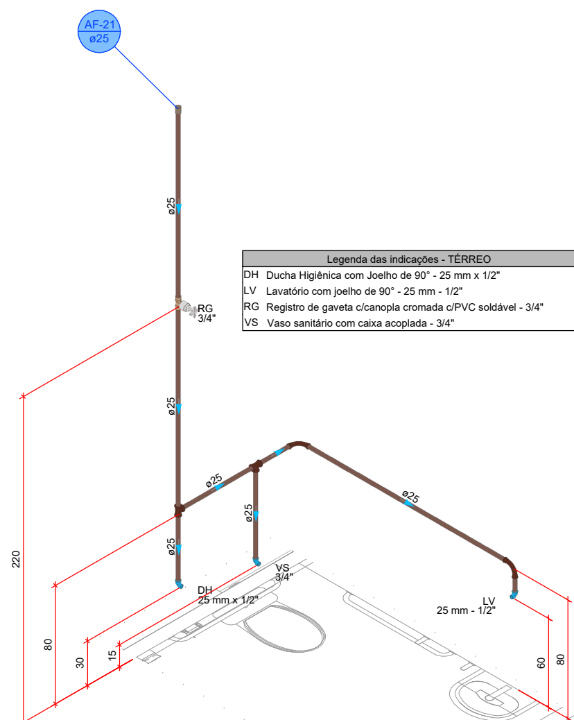
DETALHE HID-16 1:25
