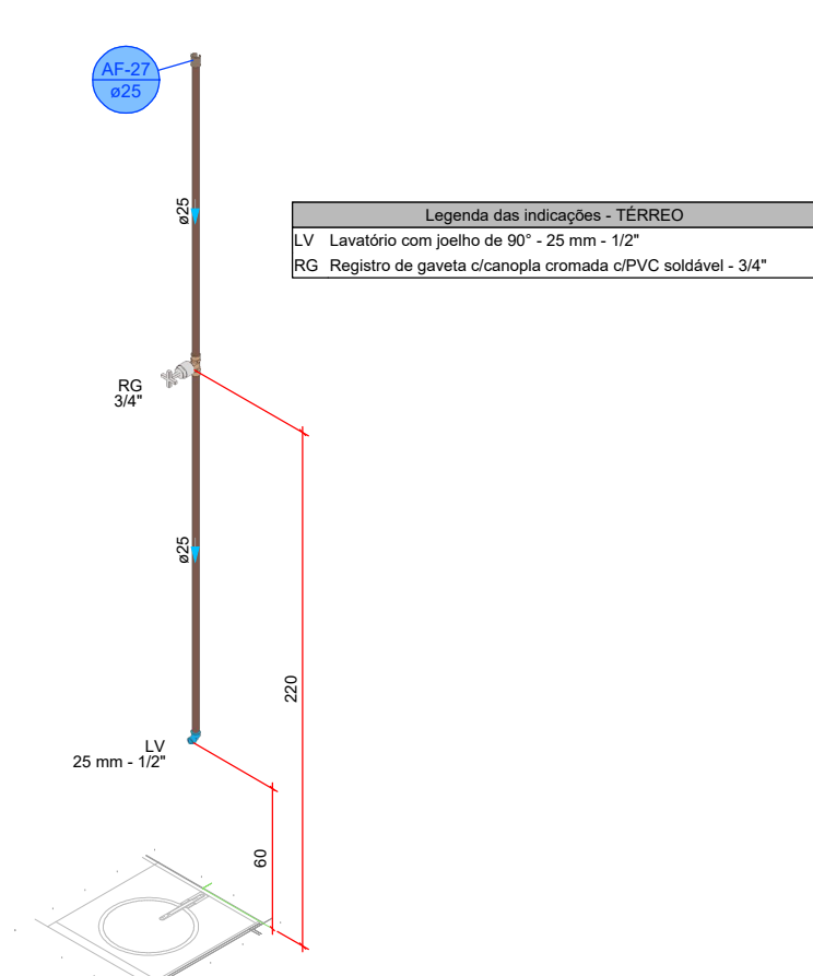
DETALHE HID-26
