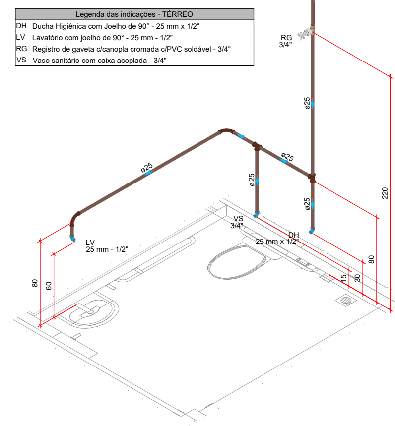
DETALHE HID-16 1:25
