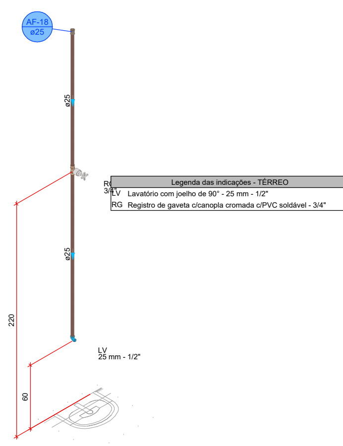
DETALHE HID-18 1:25
