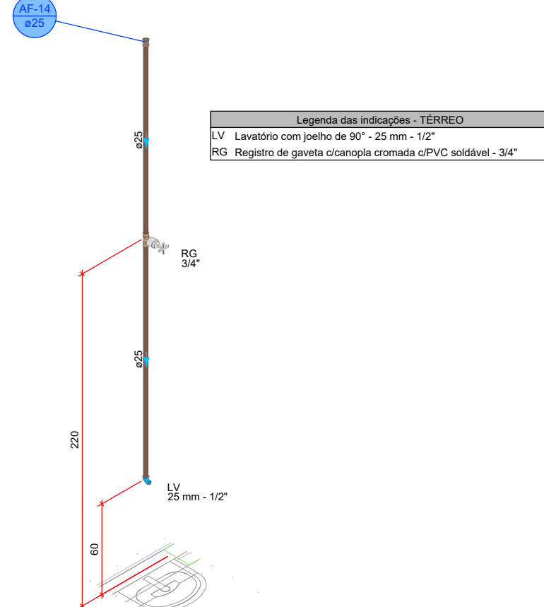
DETALHE HID-15 1:25
