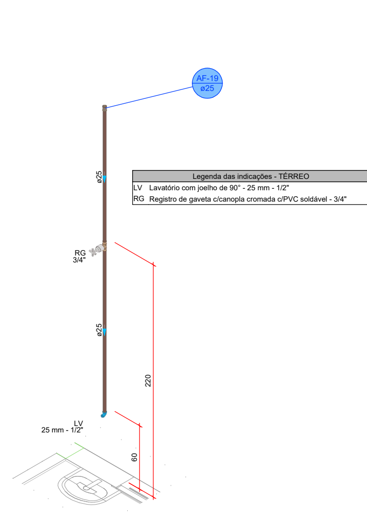
DETALHE HID-20 1:25
