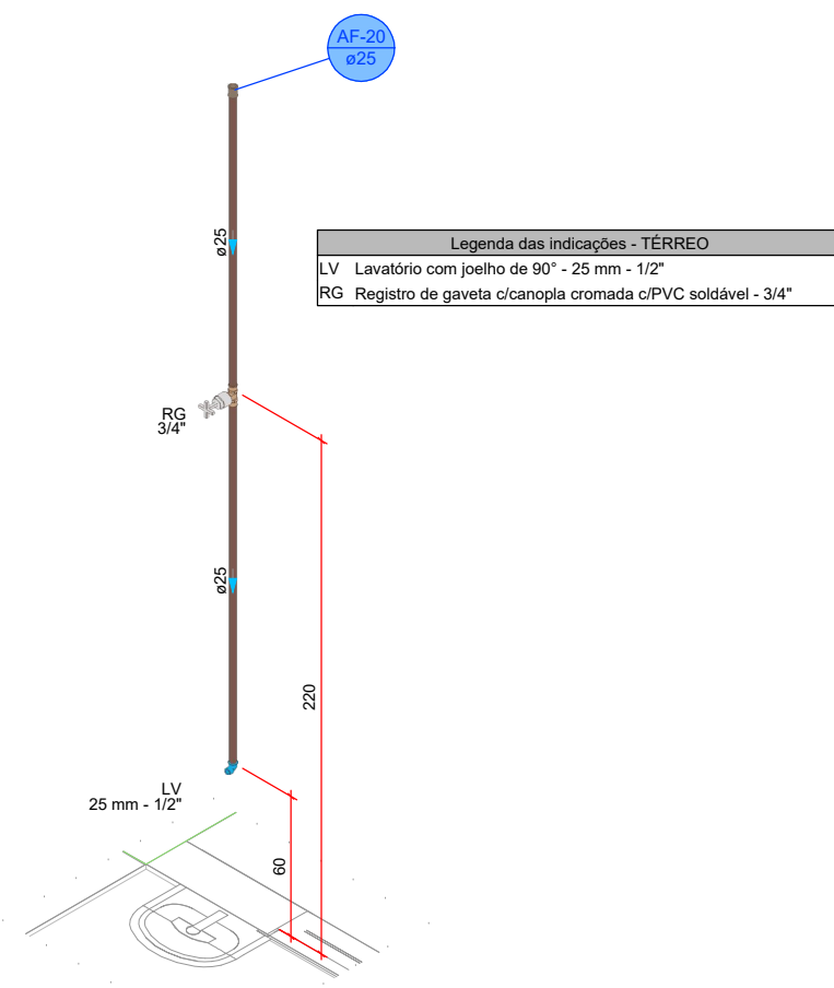
DETALHE HID-19 1:25
