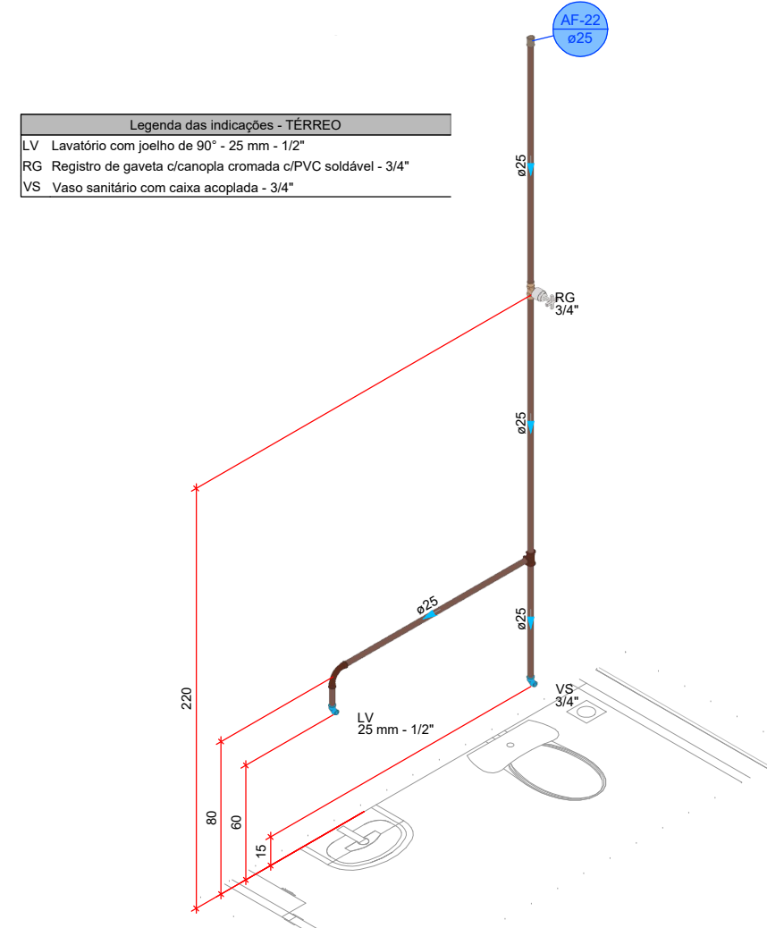
DETALHE HID-22 1:25
