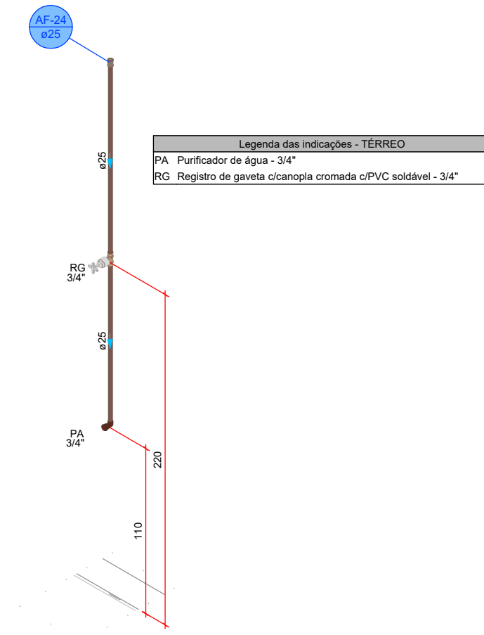
DETALHE HID-24 1:25
