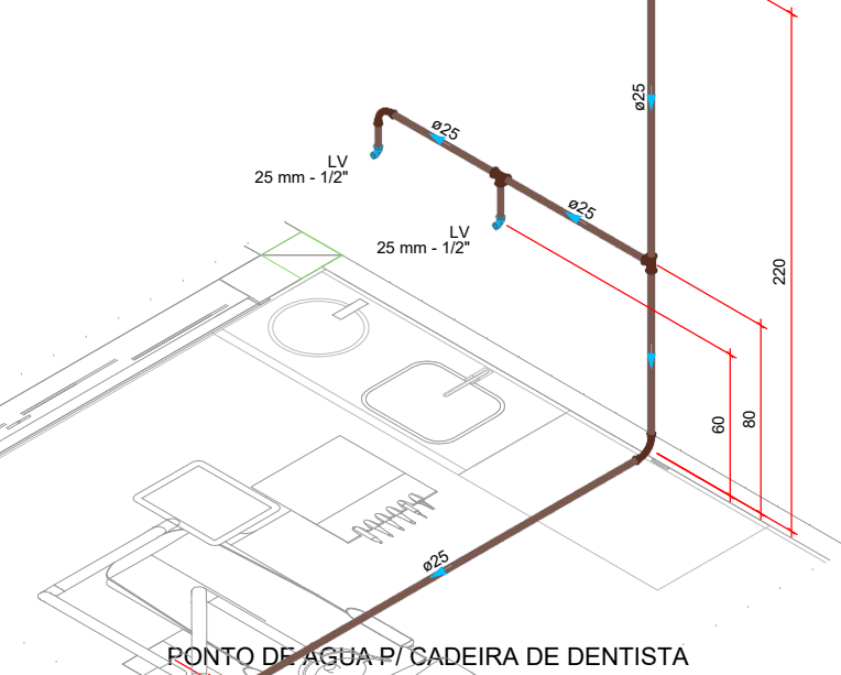
DETALHE HID-13 1/25
