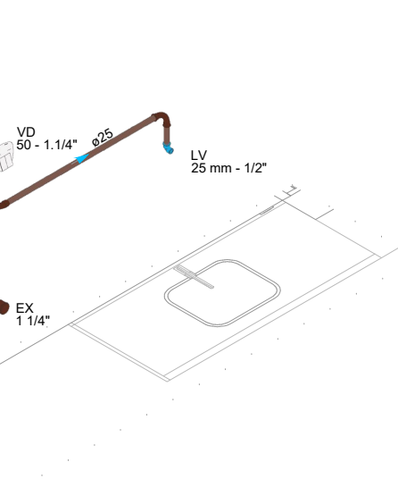
DETALHE HID-8 1/25
