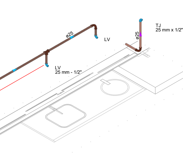
DETALHE HID-11 1/25
