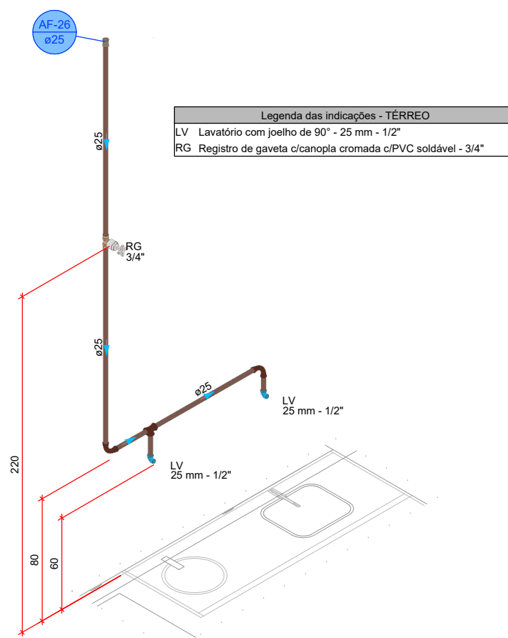
DETALHE HID-25 1:25
