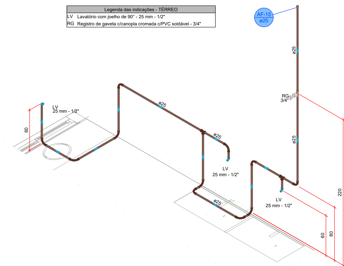
DETALHE H14 1:25
