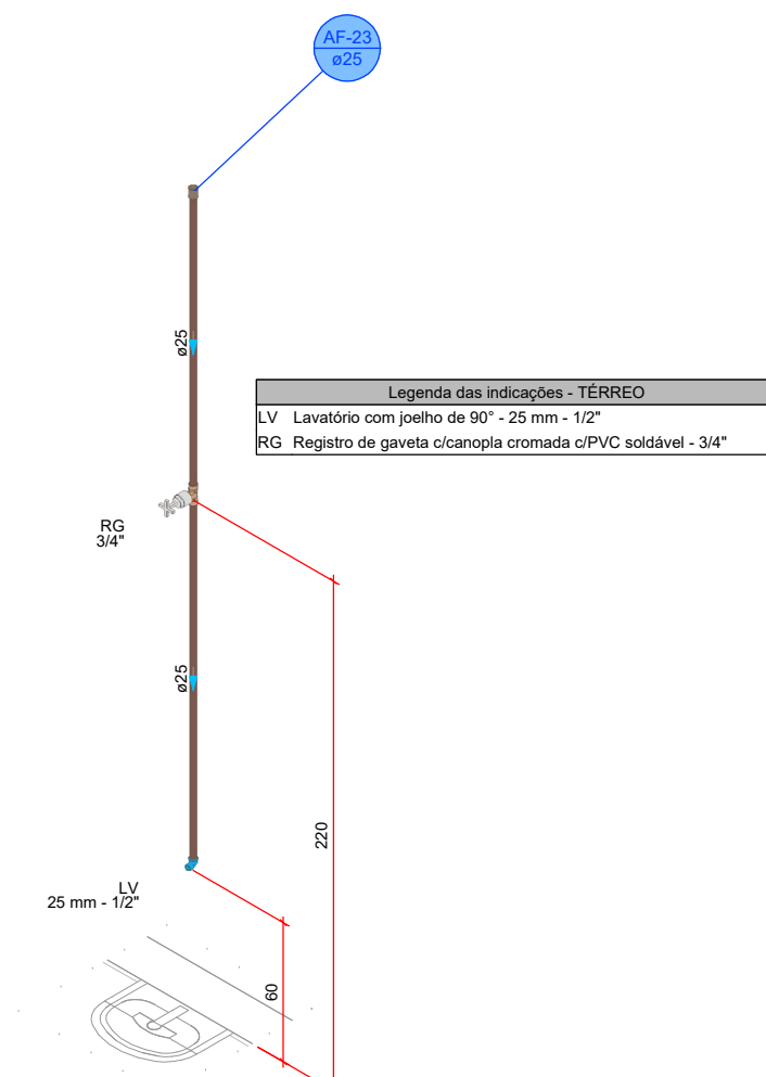
DETALHE HID-23 1:25
