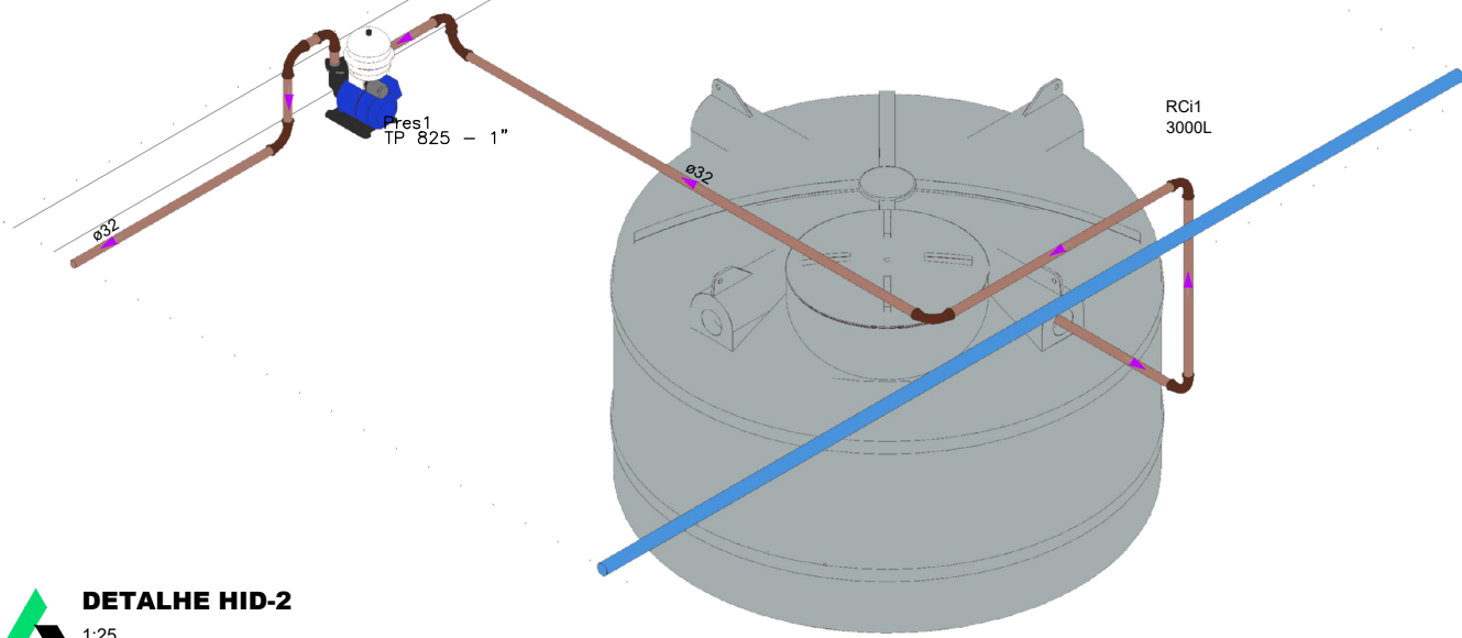
DETALHE HID-2 1/25
