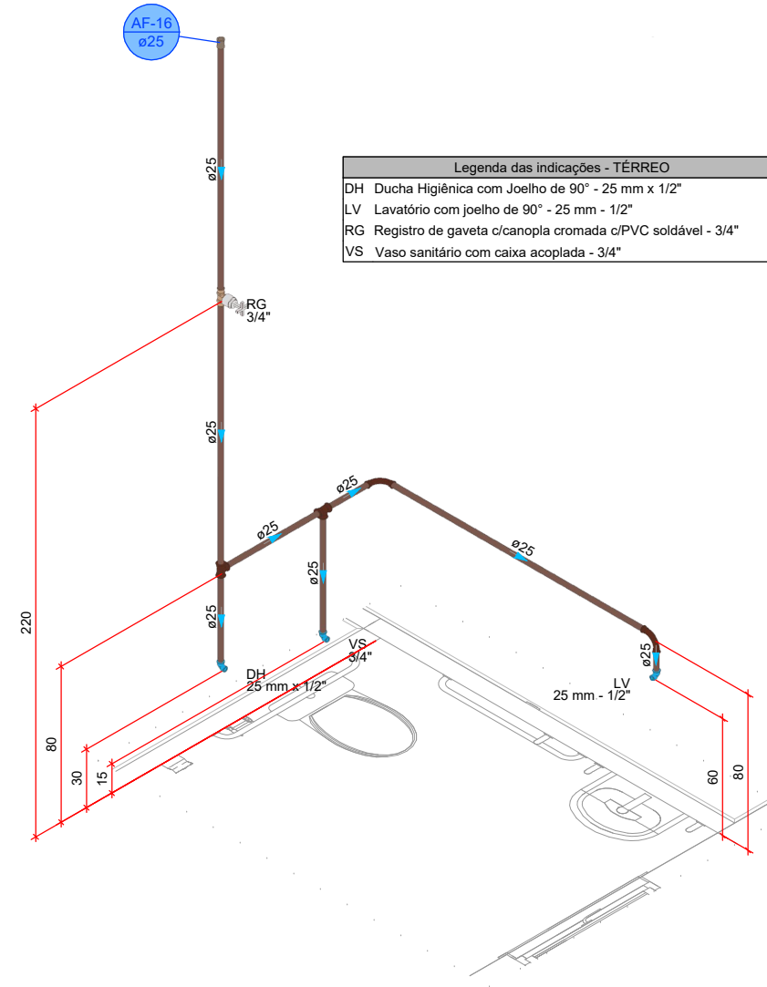
DETALHE HID-17 1:25
